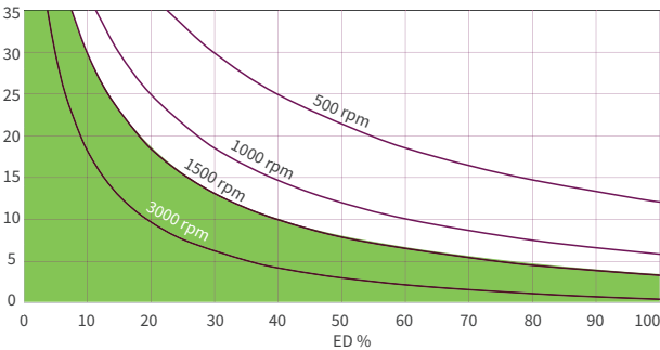
ZE-H 50 кН смазка маслом, пер. отношение 7:1
