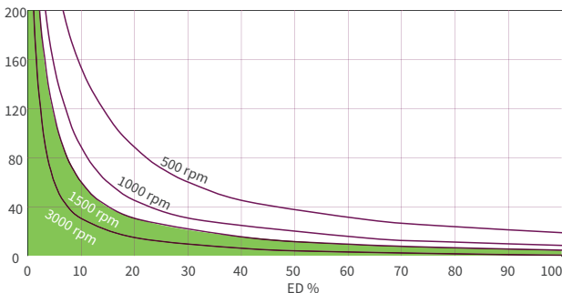
ZE-H 200 кН смазка маслом, пер. отношение 8:1
