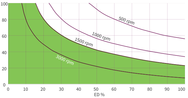
ZE-H 150 кН смазка маслом, пер. отношение 36:1
