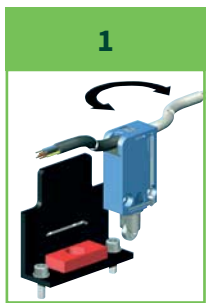
1 Выход кабеля меняется на 180°
