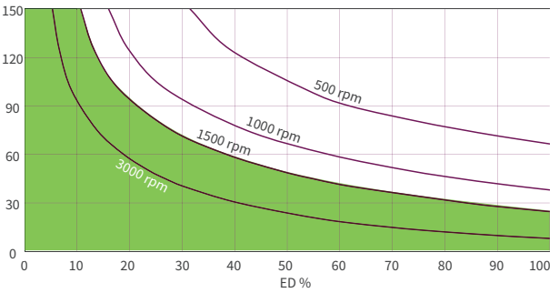
ZE-H 200 кН смазка маслом, пер. отношение 24:1
