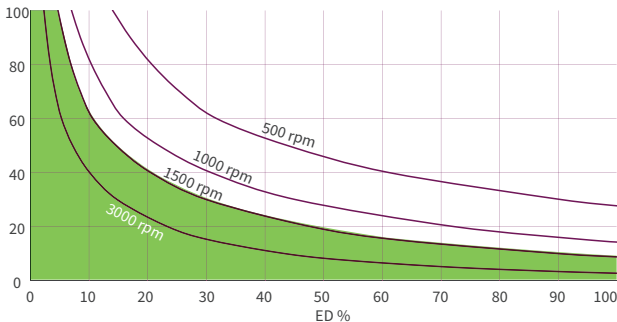
ZE-H 150 кН смазка маслом, пер. отношение 9:1
