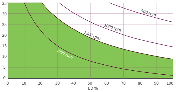
ZE-H 50 кН смазка маслом, пер. отношение 28:1
