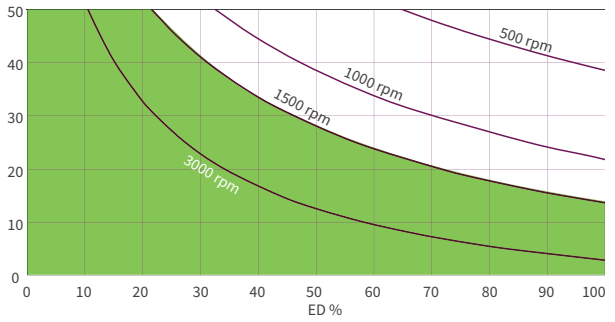
ZE-H 100 кН смазка маслом, пер. отношение 36:1
