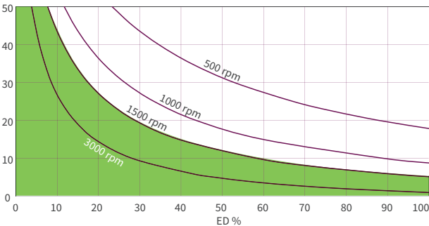
ZE-H 100 кН смазка маслом, пер. отношение 9:1
