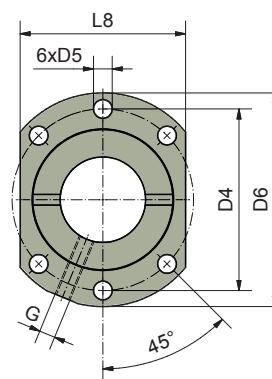
Крепежные отверстия: исполнение 1 по DIN 69051
